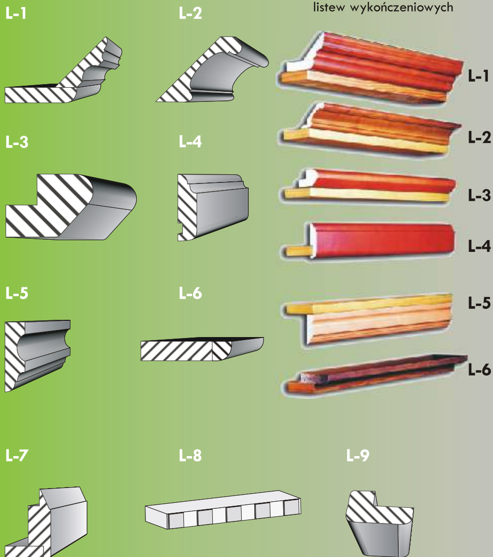
Przykłady mocowania listew wykończeniowych
